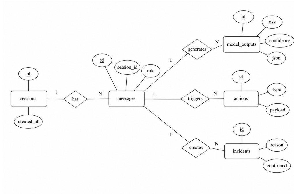
Figure 3.2: ER diagram
